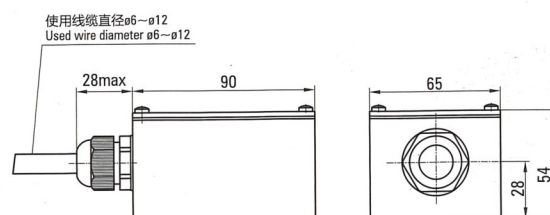
型号Model:ZDTC 安装尺寸□80mm、□90mm、□104mm 电动机Motor with the flame size of □80mm、□90mm、□104mm
